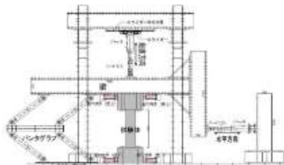
図2 多目的載荷装置全体図
