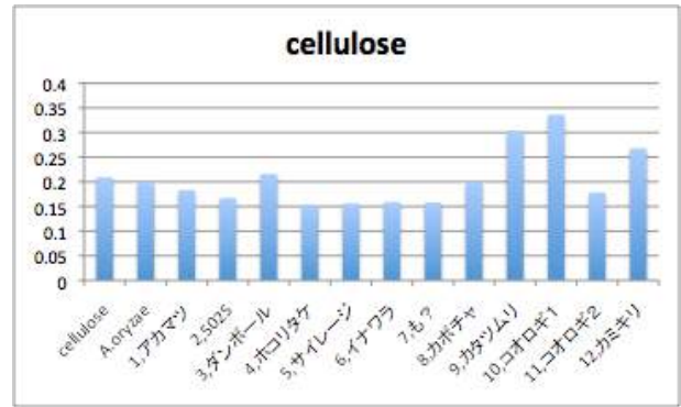
図 19 ツアペドックス・セルロース培地で各菌株を培養した培養液の 490nm 吸光度
