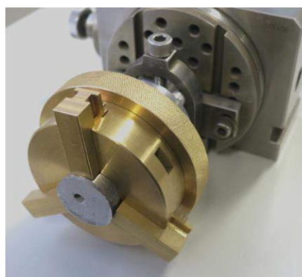
図7 割出盤に取り付けたスクロールチャック
