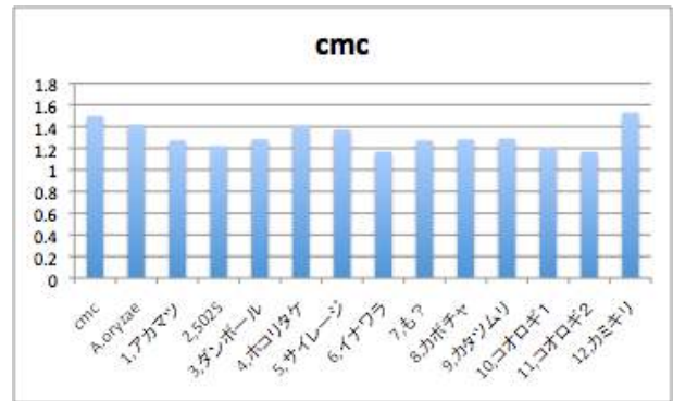
図 20 ツアペドックス・CMC 培地で各菌株を培養した培養液の 490nm 吸光度。
