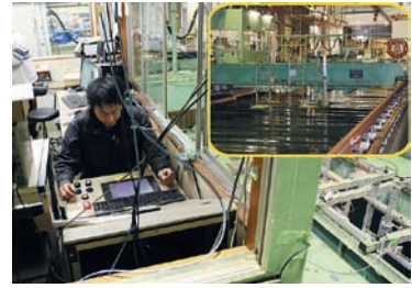
水槽実験の実施：大型水槽曳航電車
