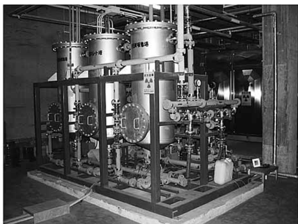
図 2. 排水設備
