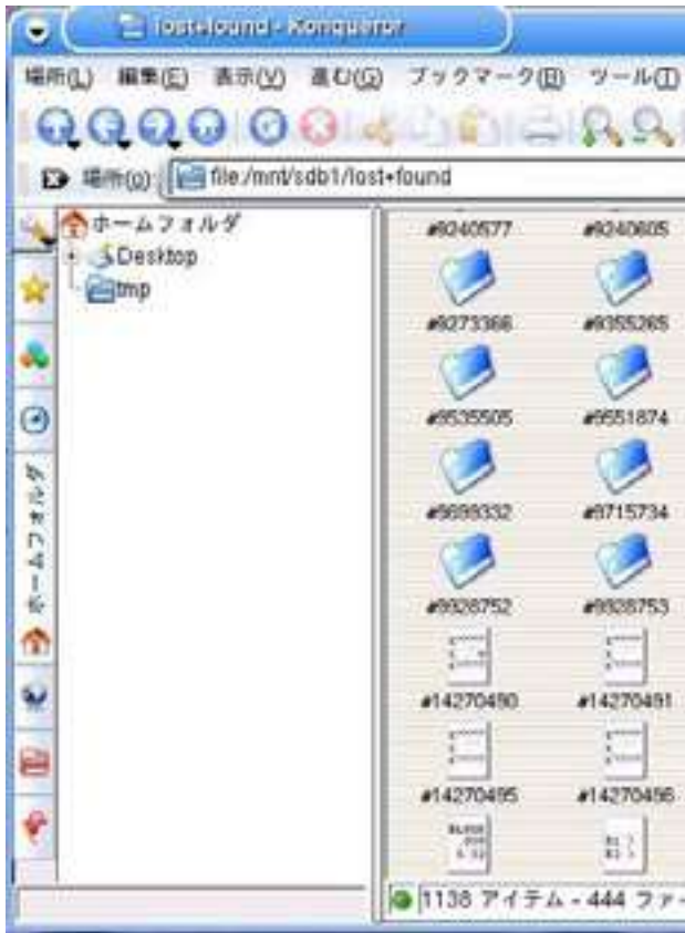
図 6 lost+found の中身
